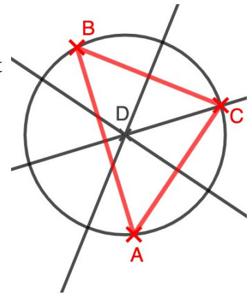
Un triangle avec ses trois médiatrices et son cercle circonscrit
