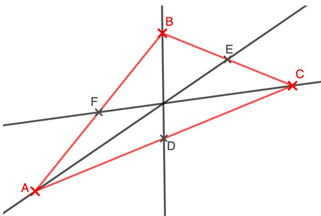
un triangle et ses trois médianes
