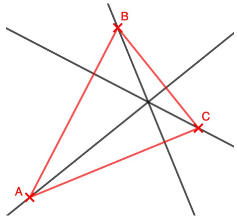
un triangle et ses trois hauteurs
