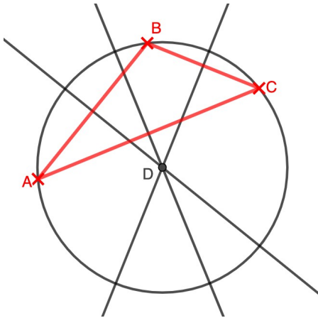
Un triangle avec ses trois médiatrices et son cercle circonscrit
