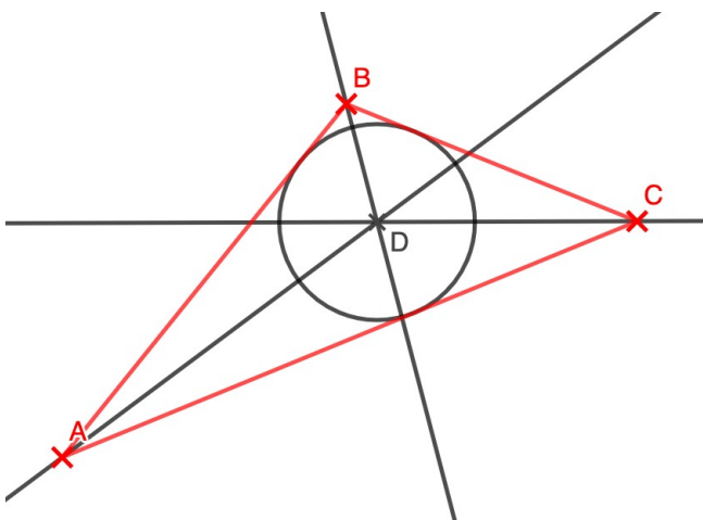
un triangle, ses trois bissectrices et son cercle inscrit
