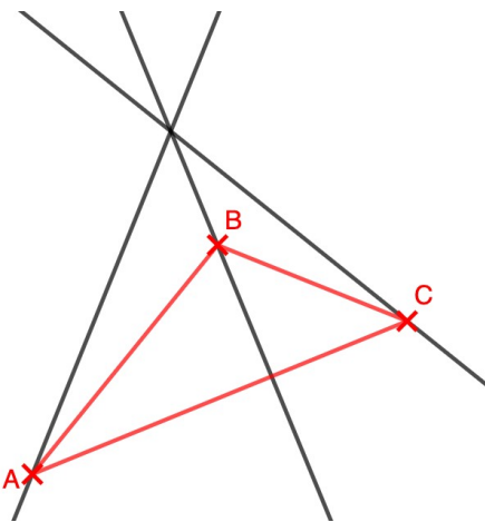
un triangle et ses trois hauteurs
